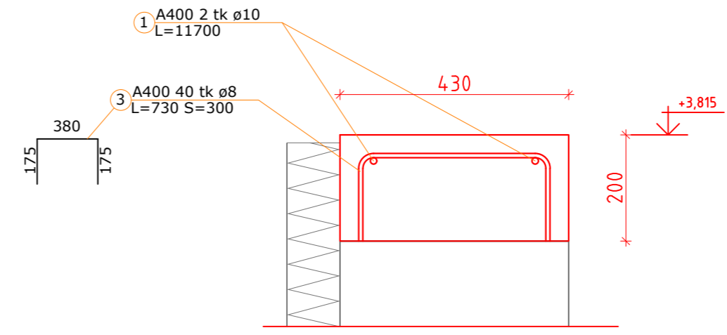
LÕIGE 1-1 1:10
