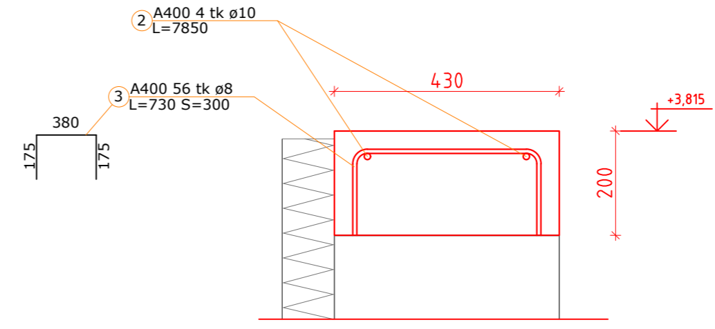
LÕIGE 2-2 1:10
