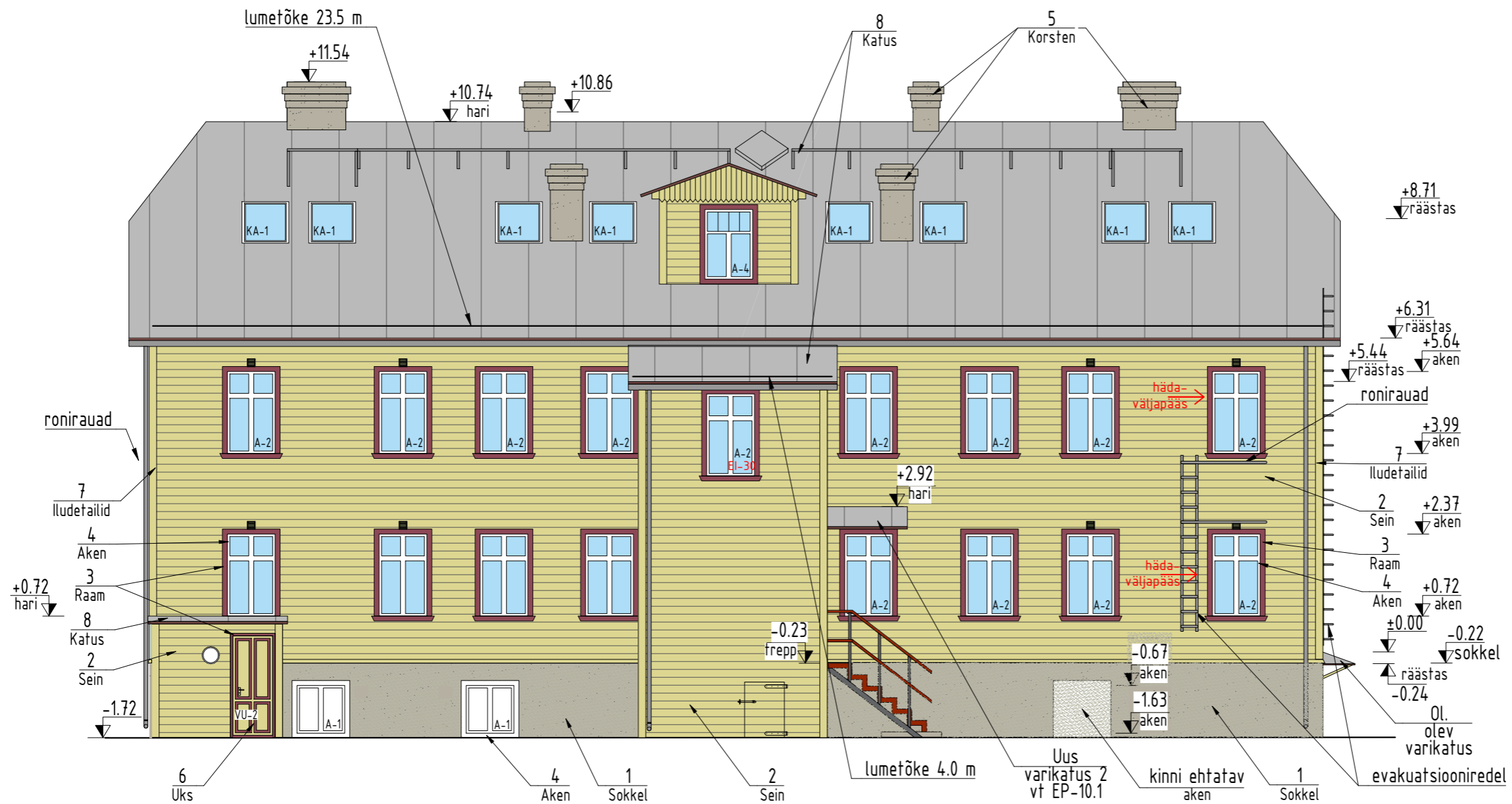
Välisvoodrilaua profiil
