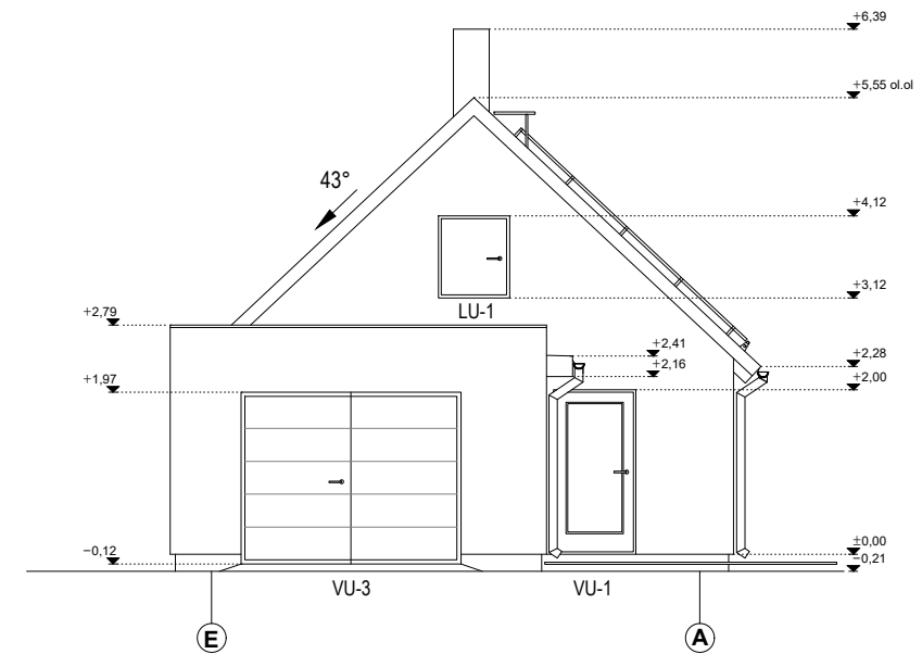
VAADE D M 1:100
