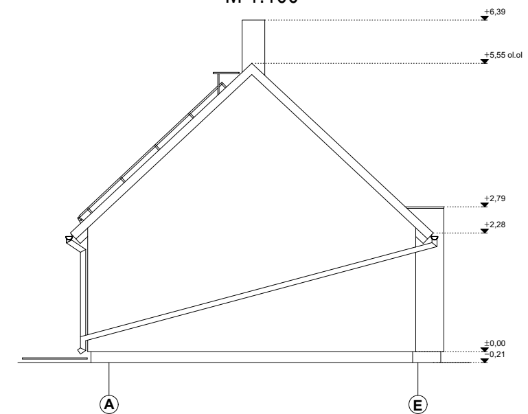
VAADE D M 1:100
