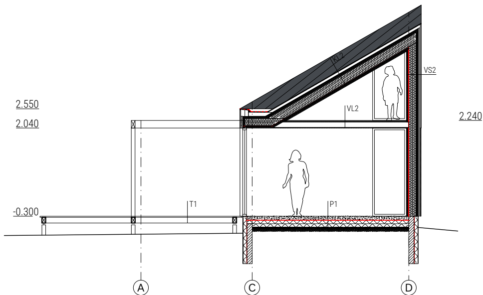
LÕIGE 2-2
