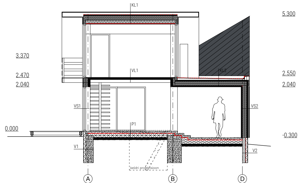
LÕIGE 1-1
