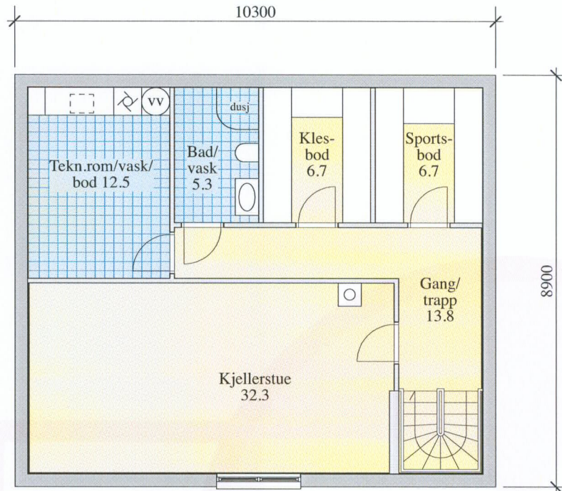
plan u.etg 81m2 BRA
