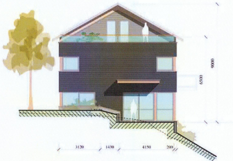
Fasade syd
