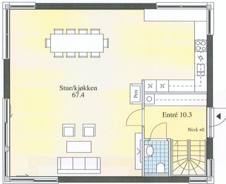
plan 1.etg 81m2 BRA
