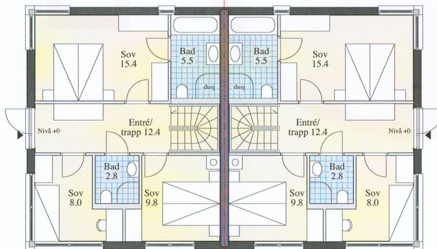
plan 1.etg 57m 2 BRA
