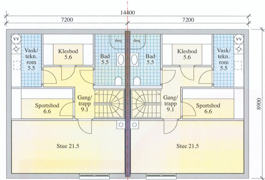
plan u.etg 56m 2 BRA
