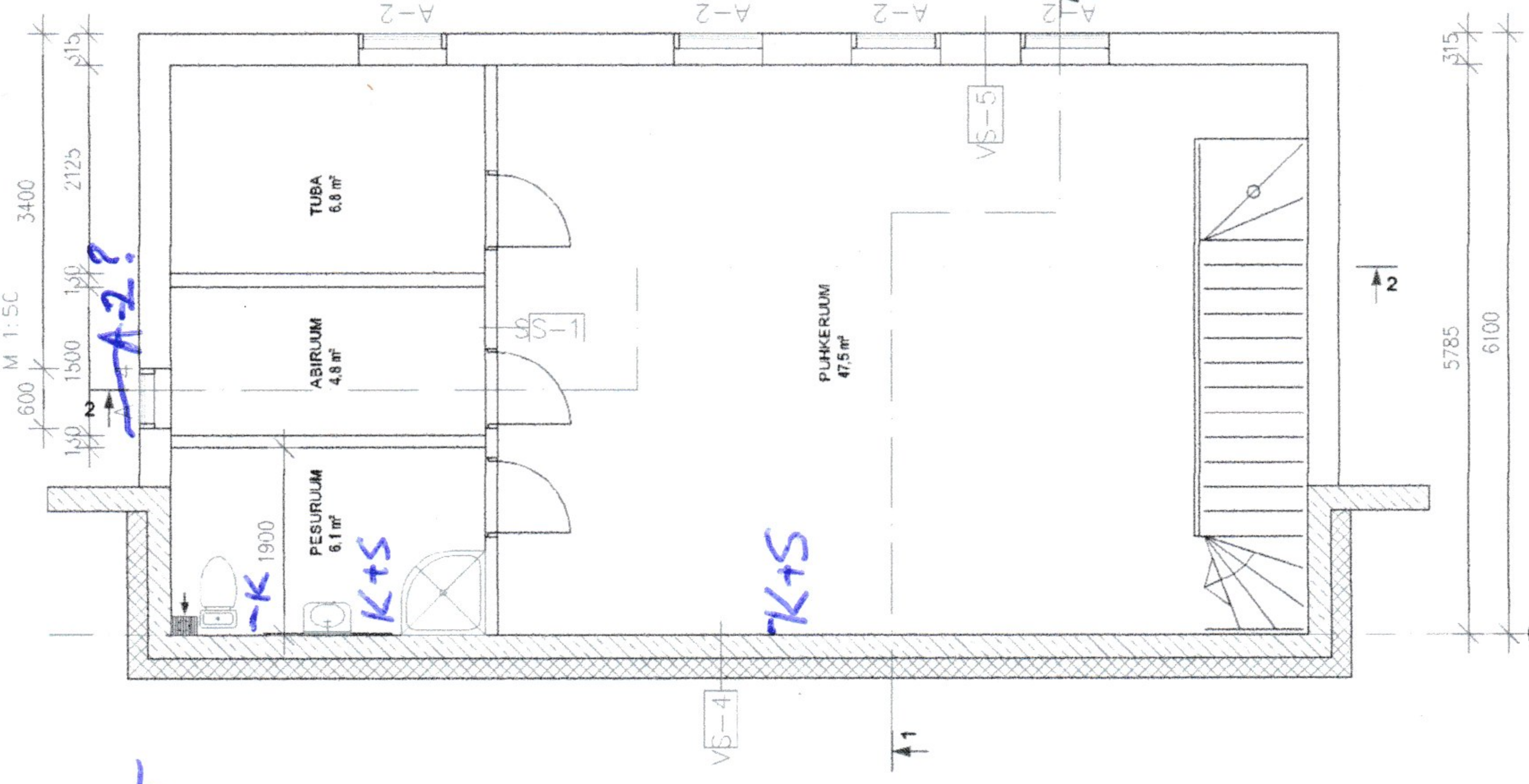
PLAAN KÕRGUSMÄRGIL +3.23
