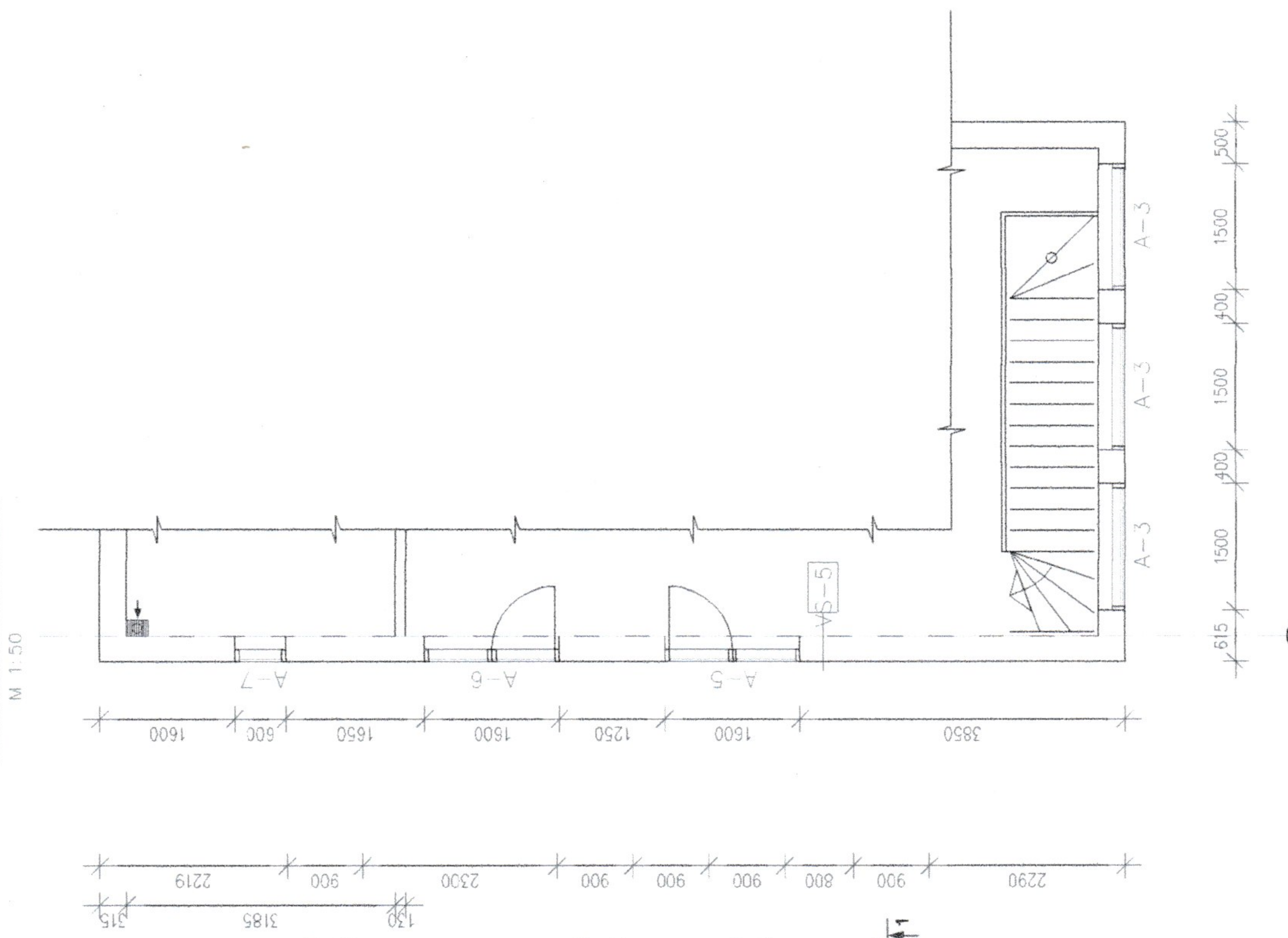
II KÕRRUSE PLAAN +3.23 SEIN TELJEL C KÕRGUSMÄRGIST +4.43
