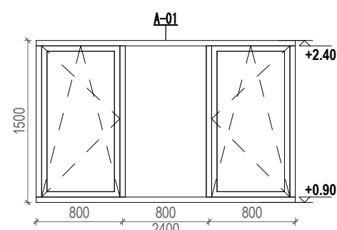
1 A-01 1 : 50
