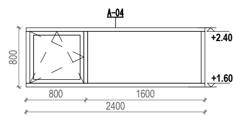
4 A-04 1 : 50
