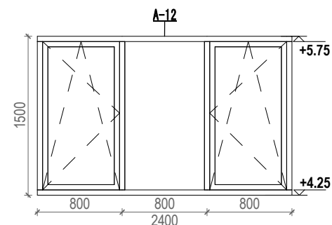
13 A-12 1 : 50
