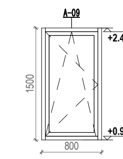
10 A-09 1 : 50
