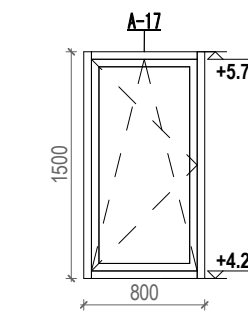
18 A-17 1 : 50
