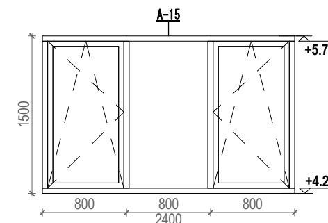
16 A-15 1 : 50
