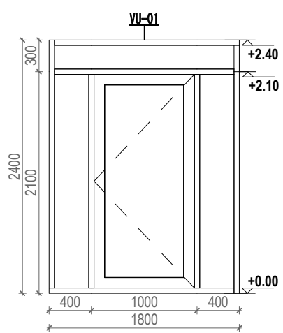
19 VU-01 1 : 50
