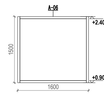
6 A-06-1 1 : 50
