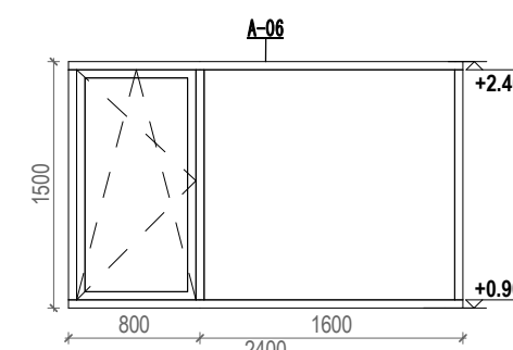
7 A-06-2 1 : 50
