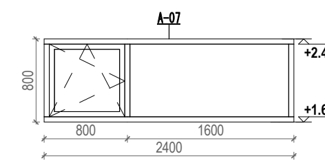
8 A-07 1 : 50
