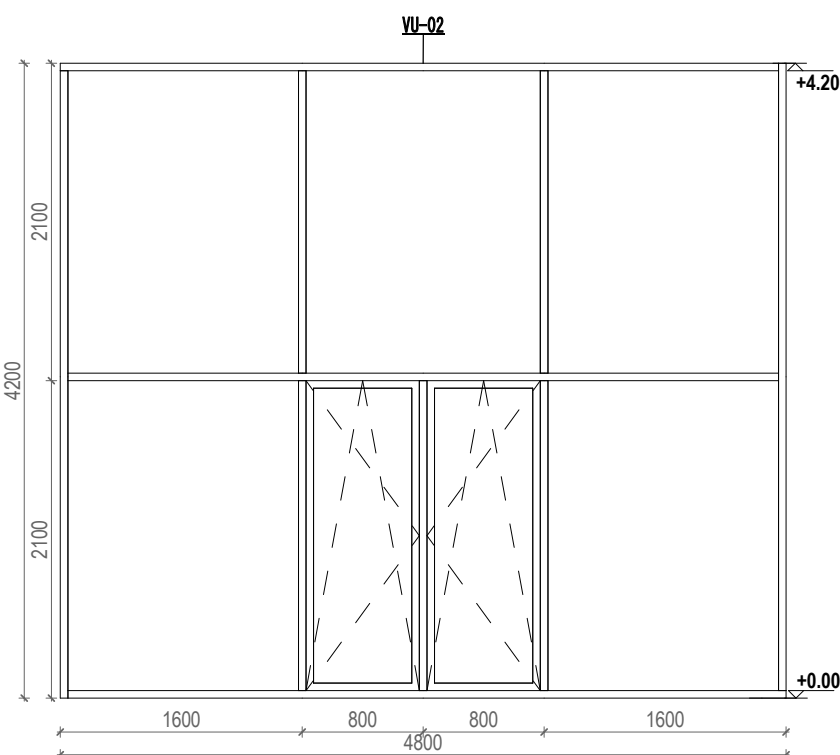
20 VU-02 1 : 50
