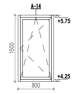
15 A-14 1 : 50
