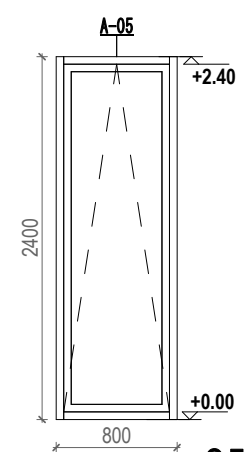
5 A-05 1 : 50
