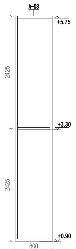
9 A-08 1 : 50
