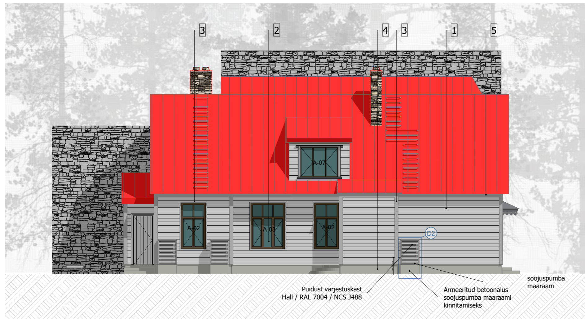
VADE PÕHJAST / M 1:100
