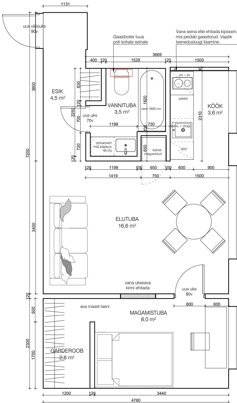
ÜMBEREHITUSE PLAAN M 1:50
