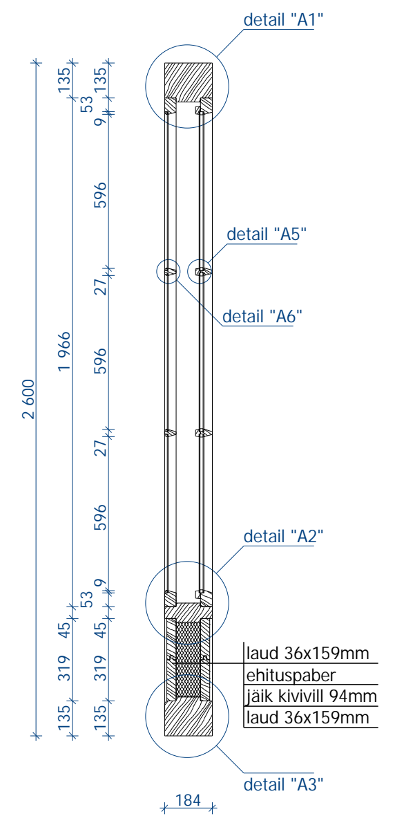
Lõige A - A
