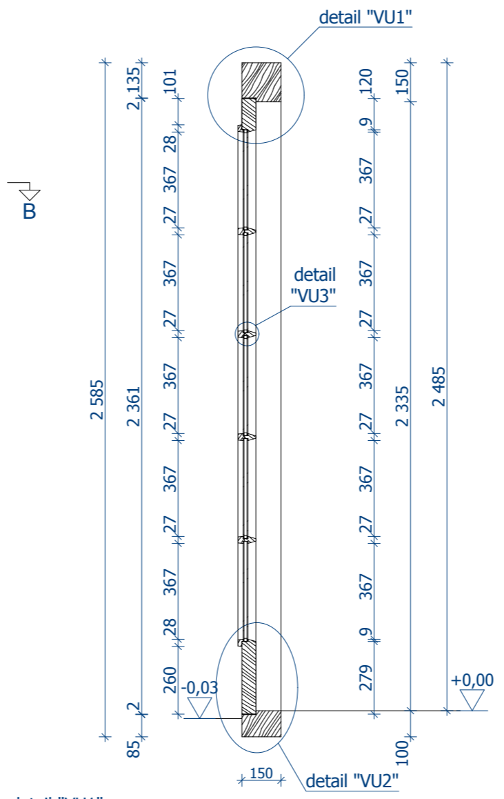
Lõige A - A
