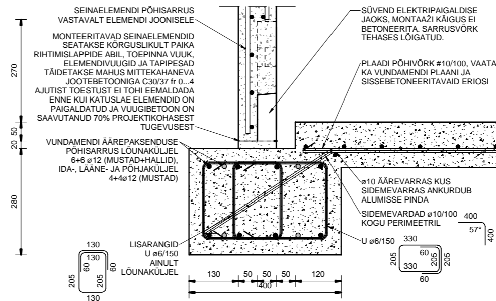
V02 Vundamendisõlm 1 : 10
