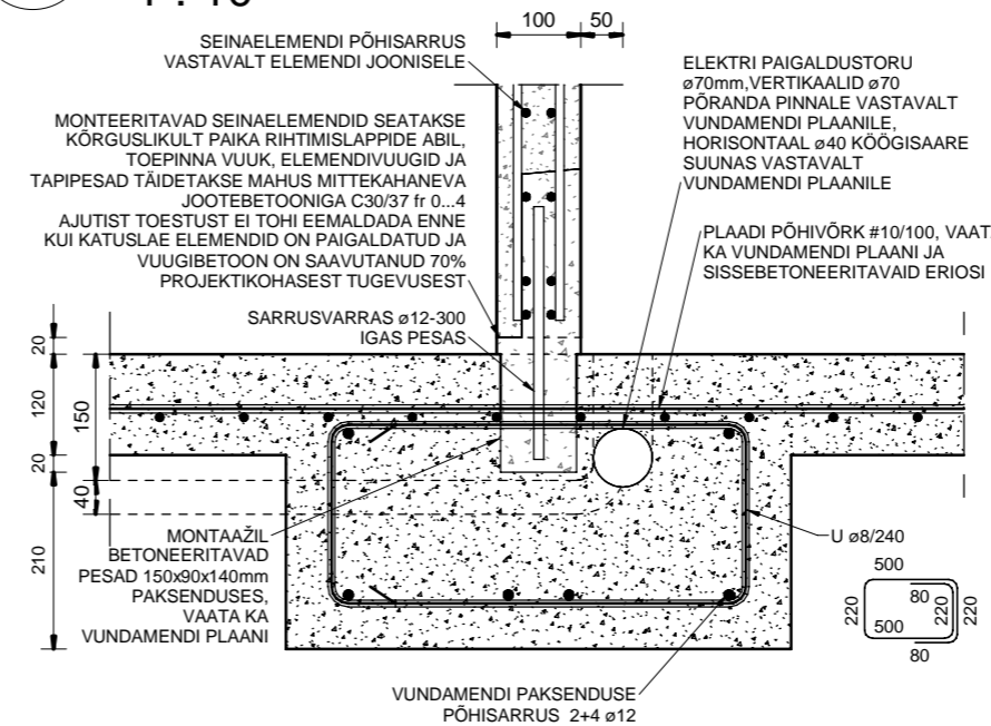
V02 Vundamendisõlm 1 : 10
