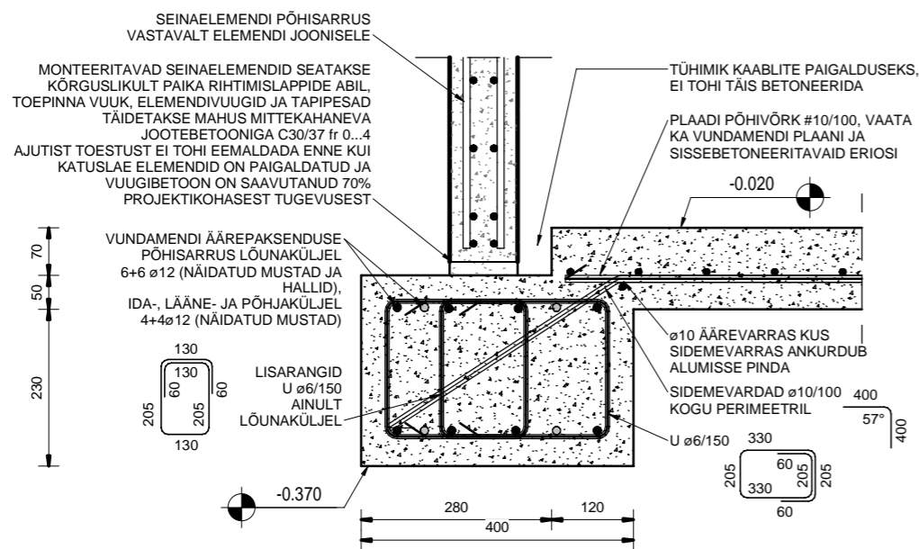
V03 Vundamendisõlm 1 : 10
