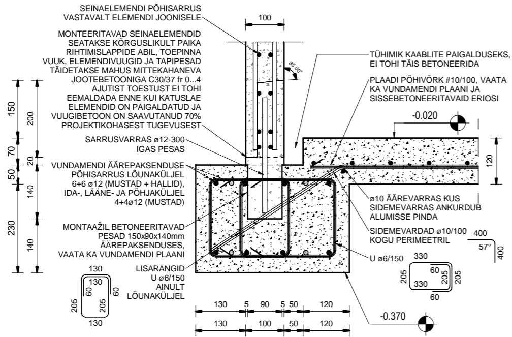
V01 Vundamendisõlm 1 : 10
