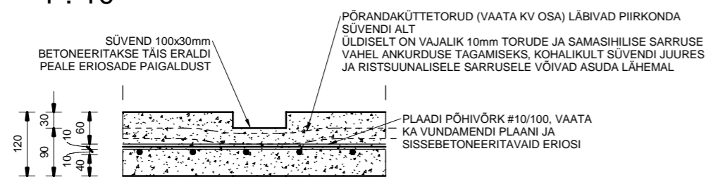
V05 Vundamendisõlm 1 : 10
