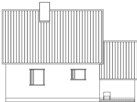
3 VAADE C 1:100
