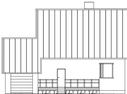
1 VAADE A 1:100
