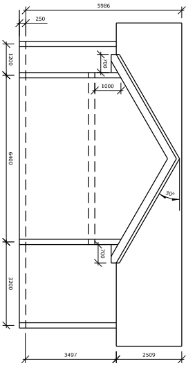
SNITT B-B
