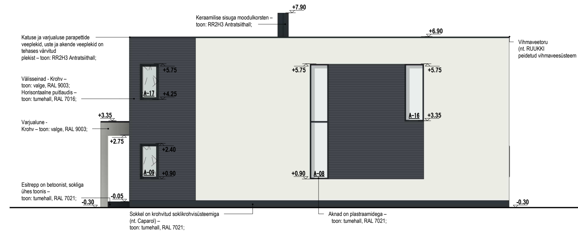
2 VADE IDAST 1 : 100
