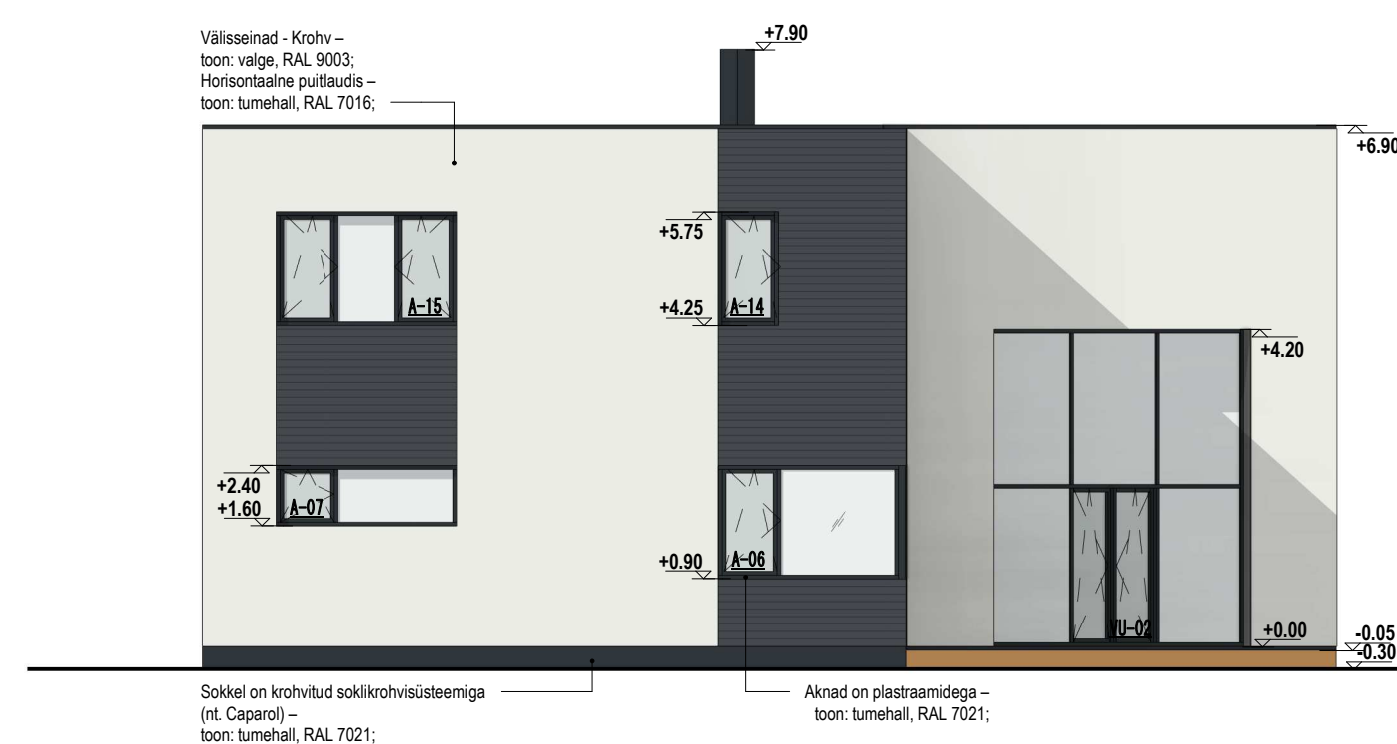
5 VADE PÕHJAST 1 : 100
