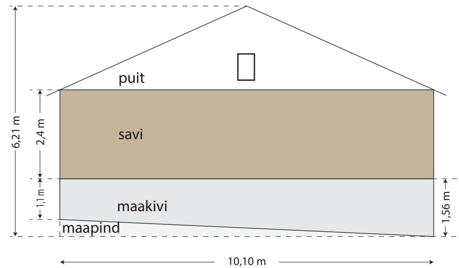
otsavaade A
