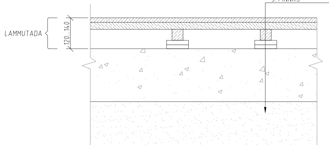
Olemasolev põrand M 1:10
