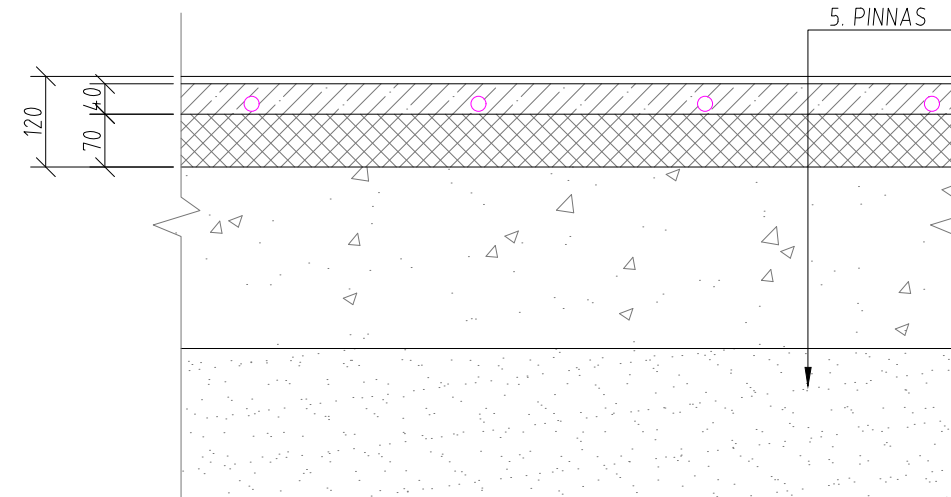
Projekteeritav põrand M 1:10
