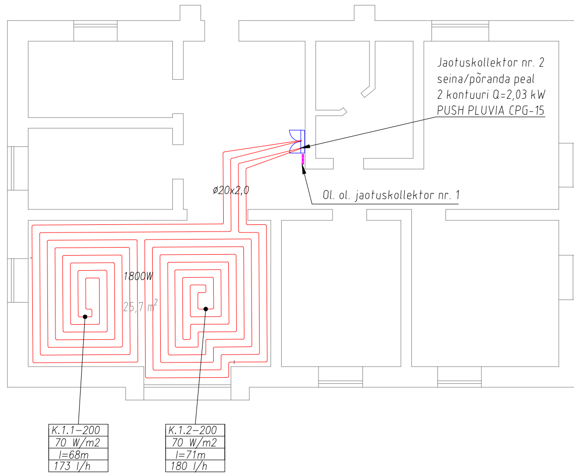
Plaan M 1:100
