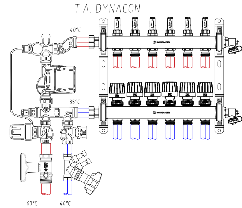
Jaotuskollektori skeem M 1:5
