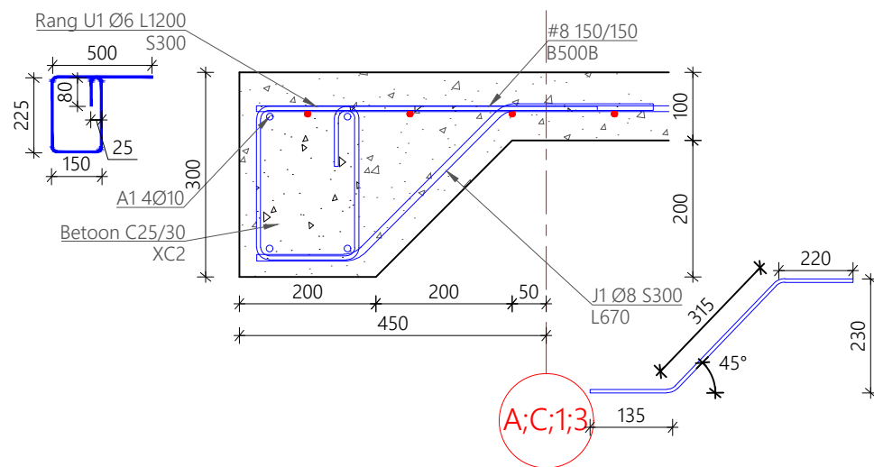
LÕIGE 2-2 M 1:10
