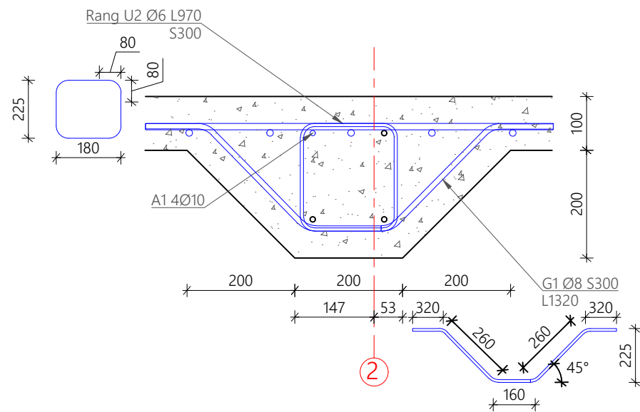
LÕIGE 2-2 M 1:10
