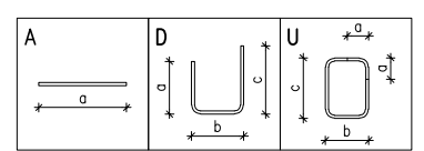
Sarruse painutustüübid
