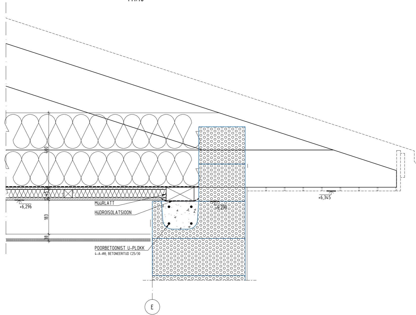
KAS 01 M1:10
