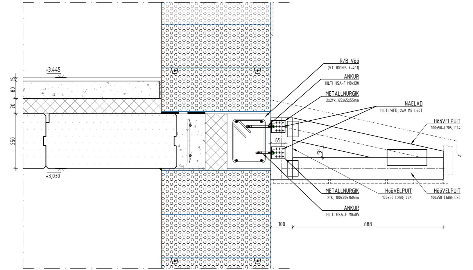
KAS 02 M1:10
