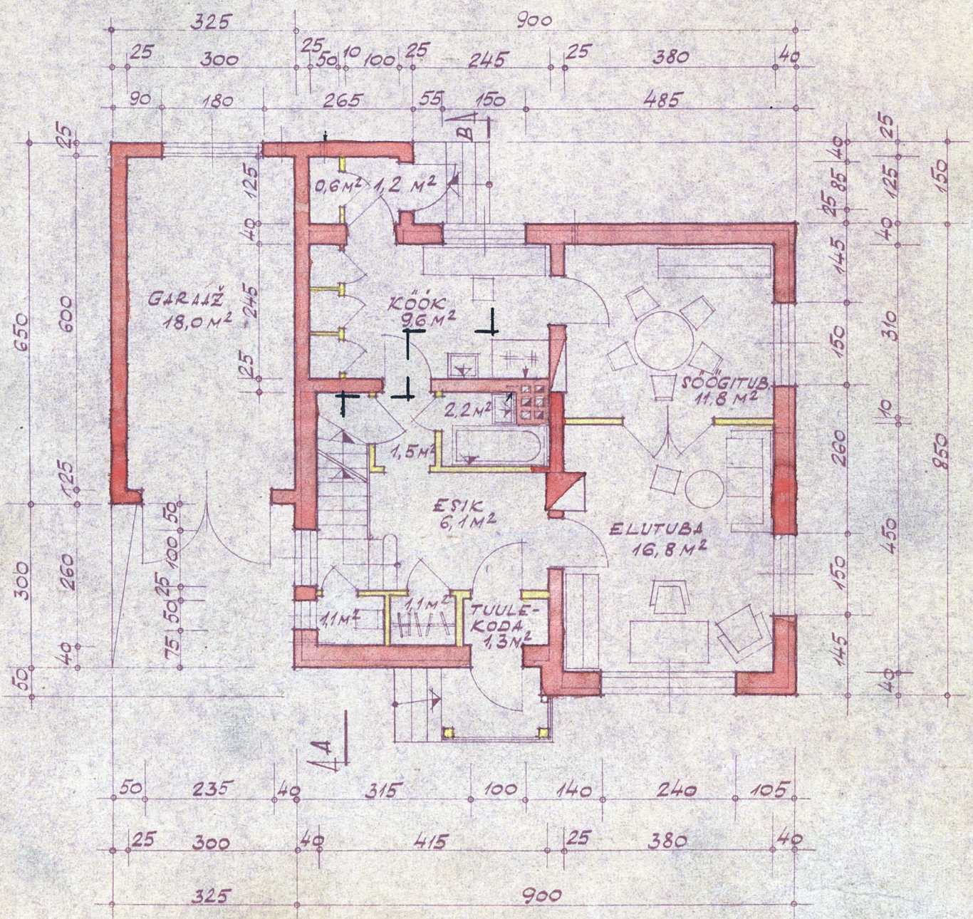
ESIMENE KORRUS M 1:100
