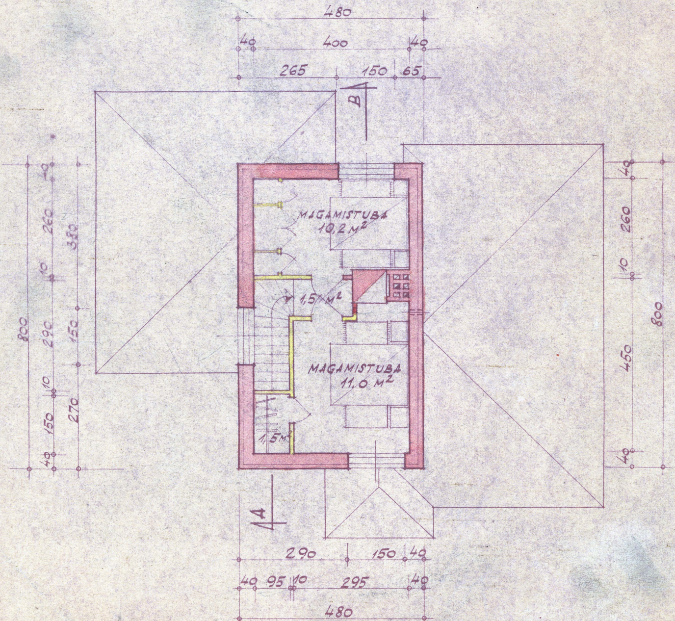
TEINE KORRUS M 1:100
