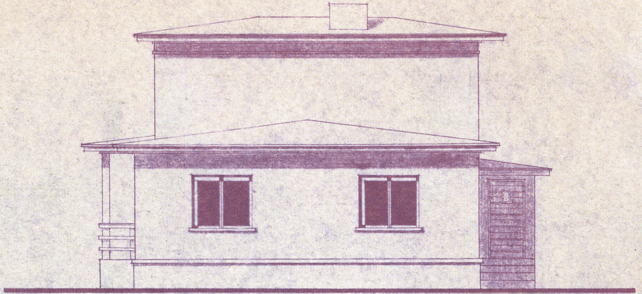
VAADE LÖUNAST 1:100
