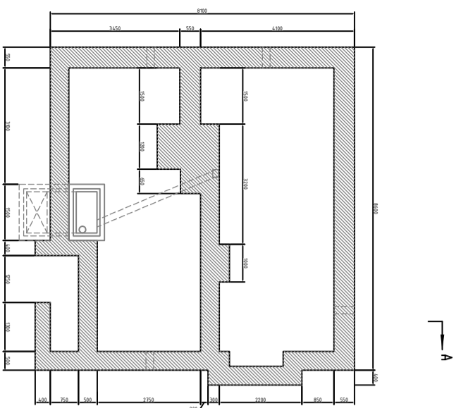
VUNDAMENT
