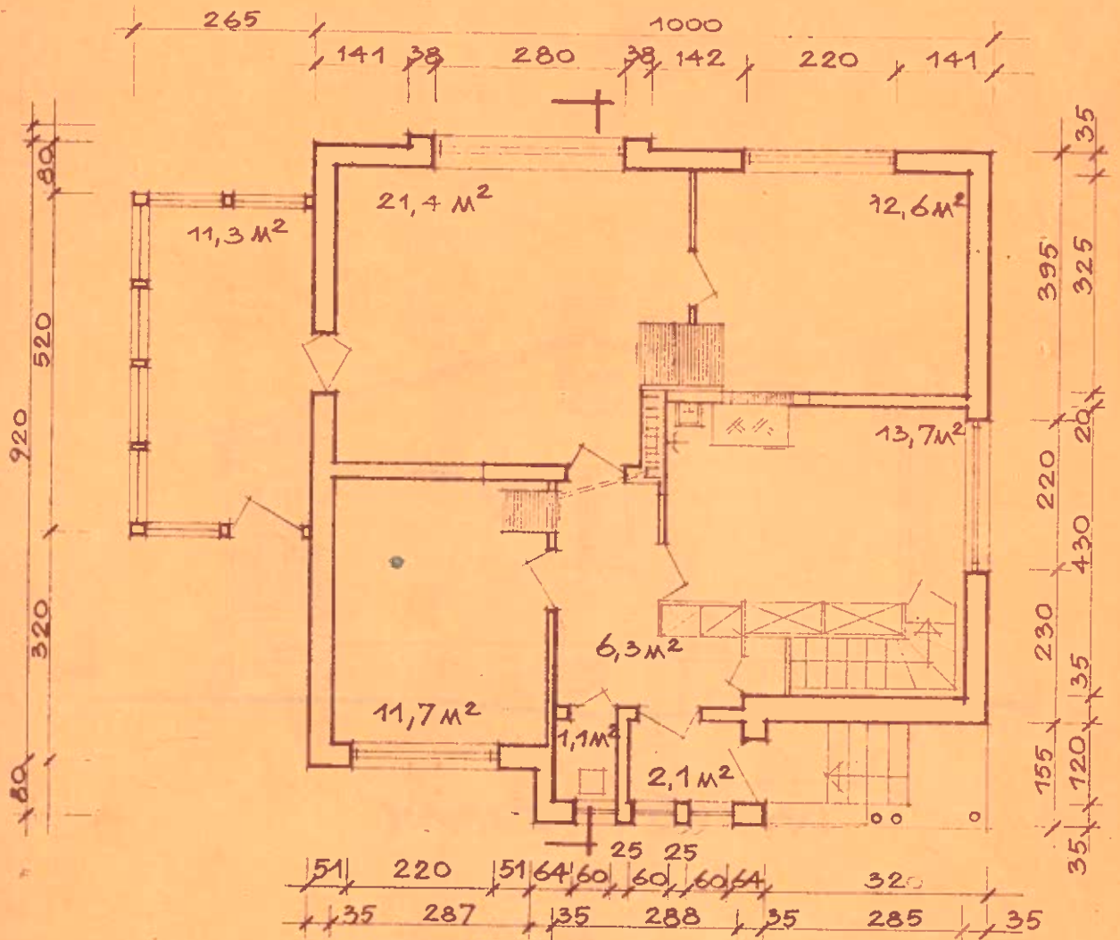
PÕHIPLAAN M 1:100
