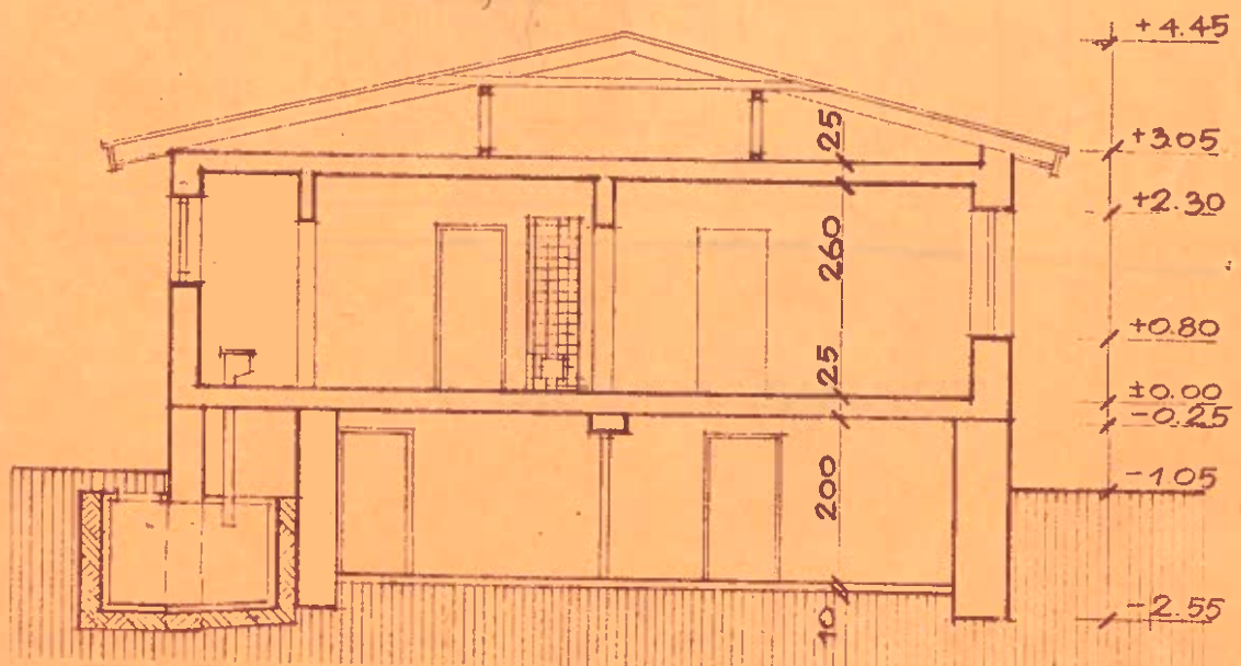
LÕIGE M 1:100
