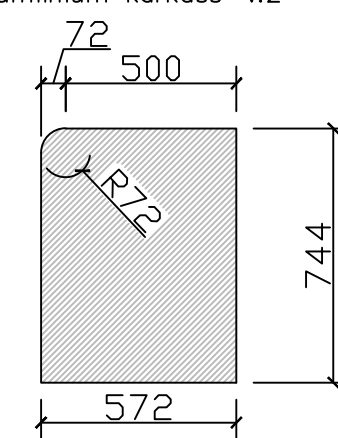
Alumiinium karkass v.2
