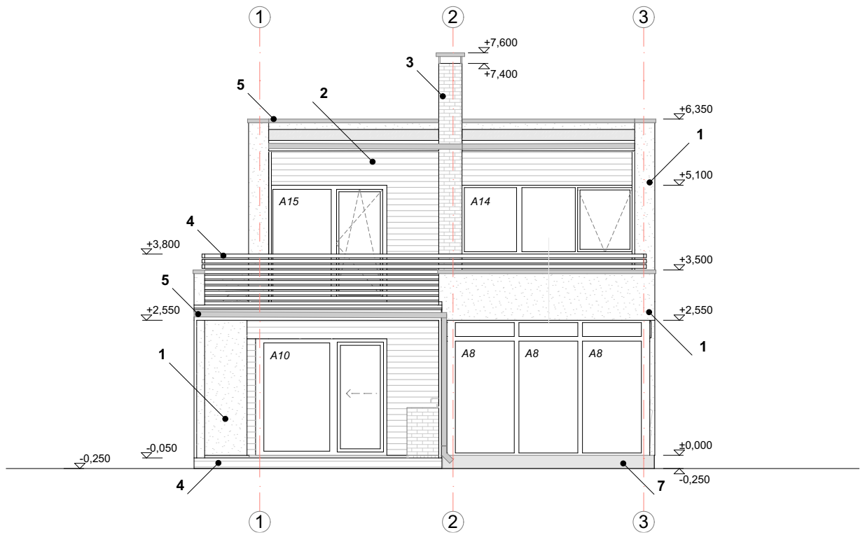
VAADE LÖUNAST
