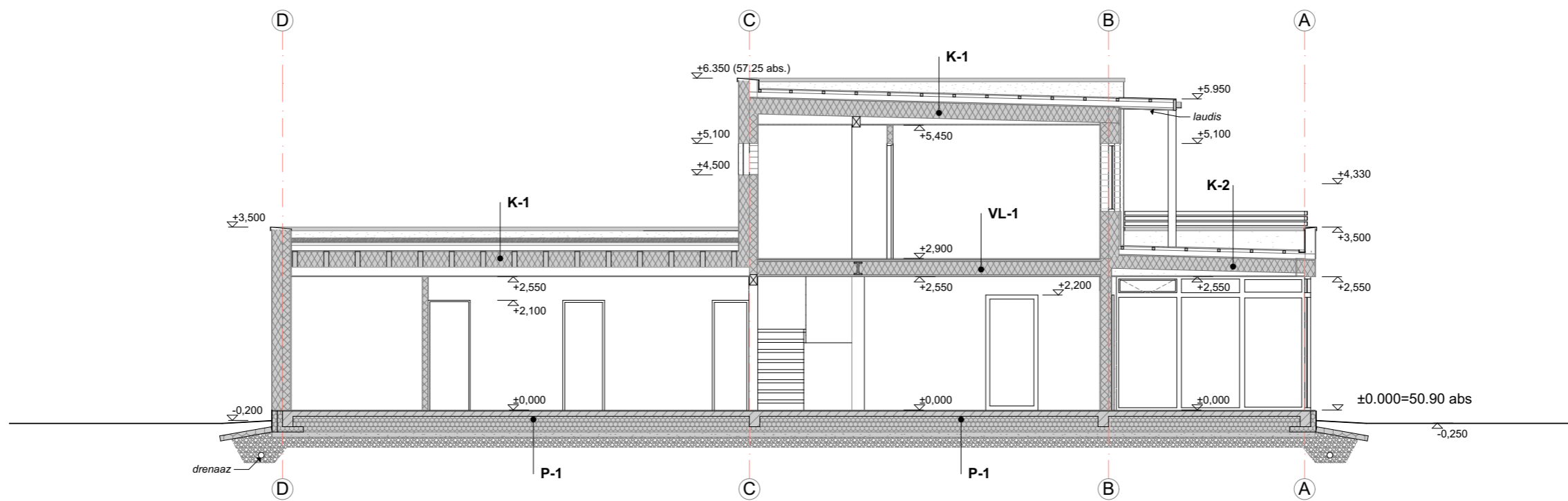
LÕIGE II-II
