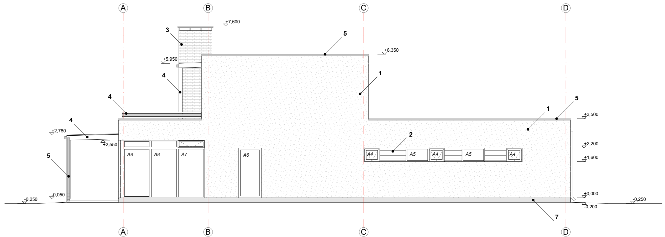
VAADE IDAST
