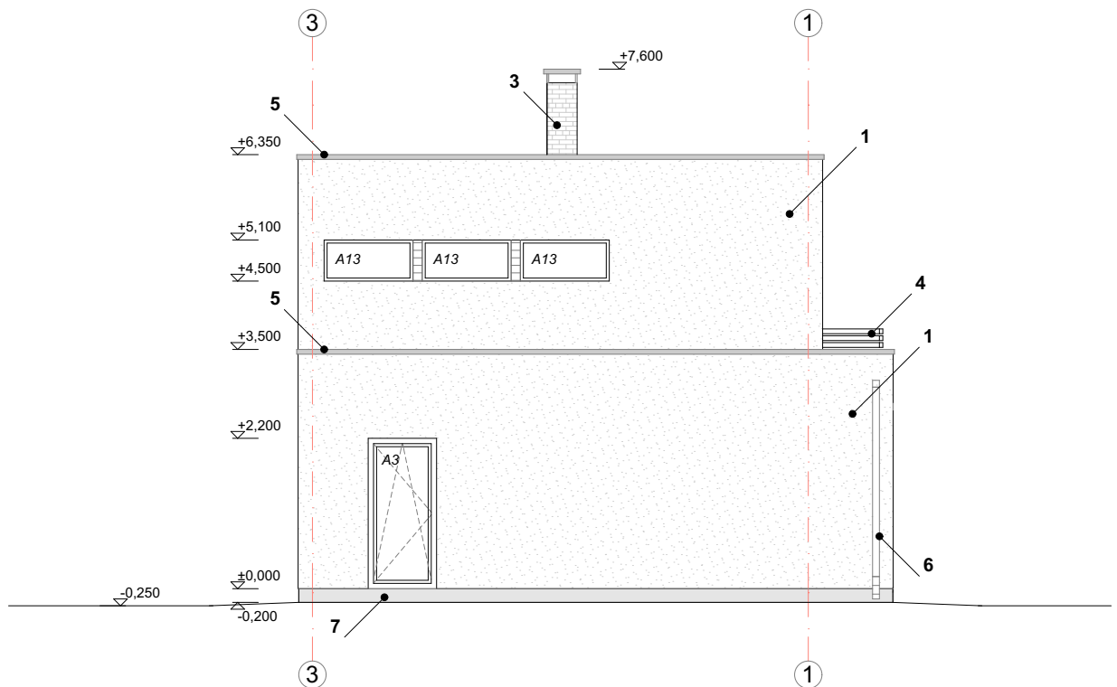
VAADE PÕHJAST
