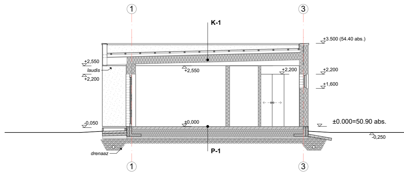
LÕIGE I-I
