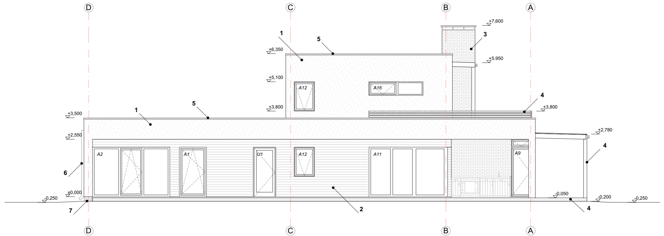
VAADE LÄÄNEST
