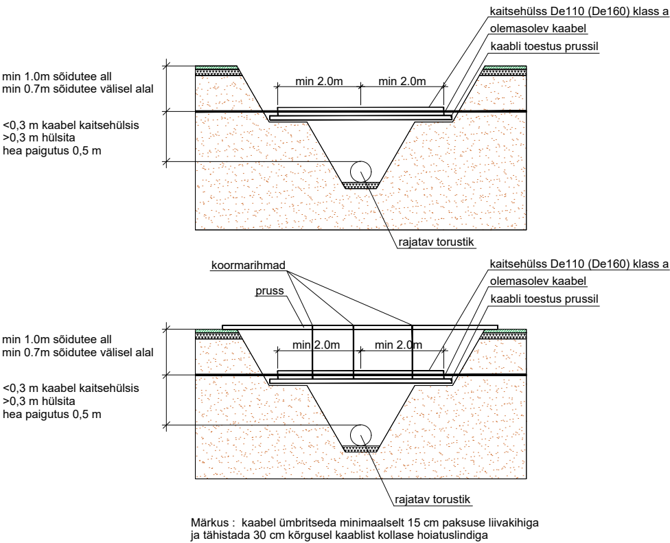
Torustiku paigaldamine ristumisel ol.ol. elektri- või sidekaabliga
