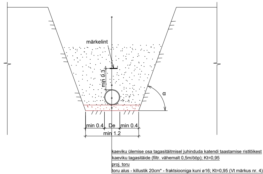
Kaeviku ristlõige Tüüp nr 2
