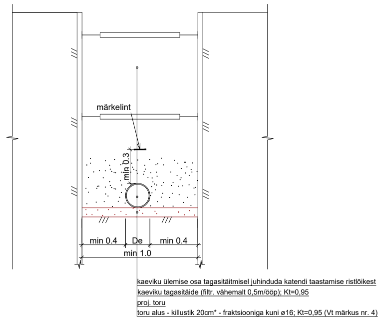
Kaeviku ristlõige Tüüp nr 2
