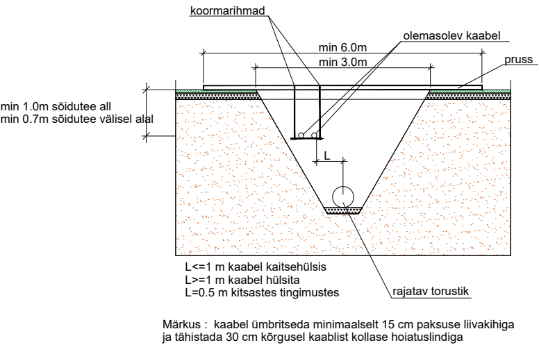
Torustiku paigaldamine paralleelsel kulgemisel ol.ol. elektri-või sidekaabliga
