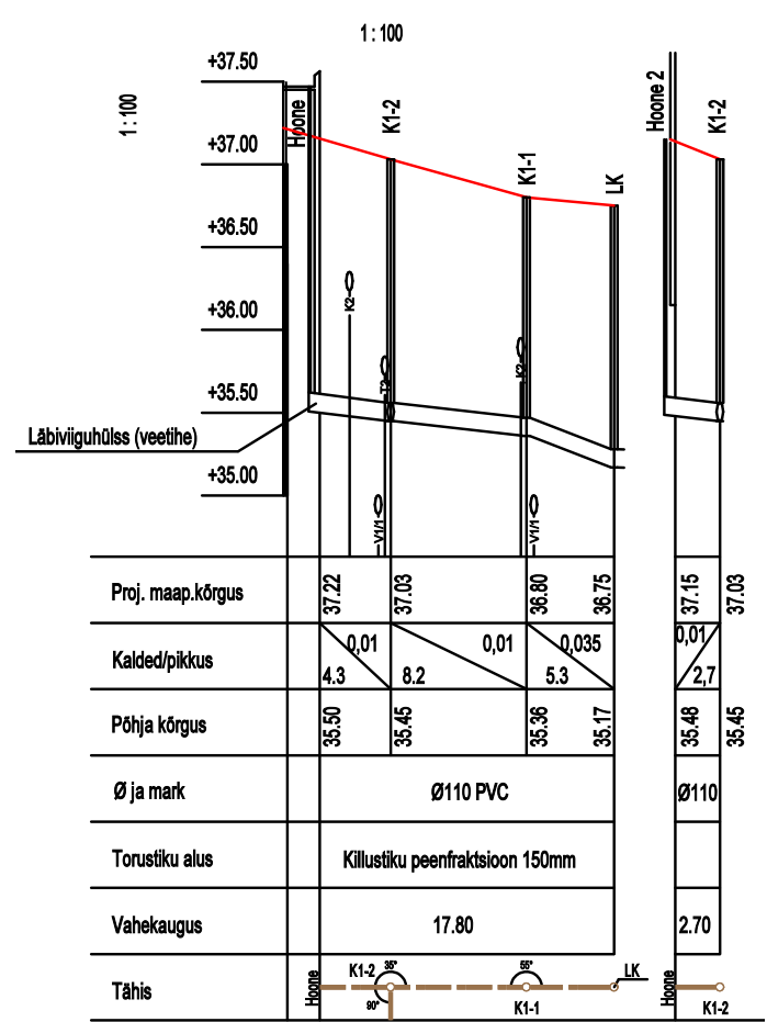
Olmekanalisatsiooni pikiprofil
