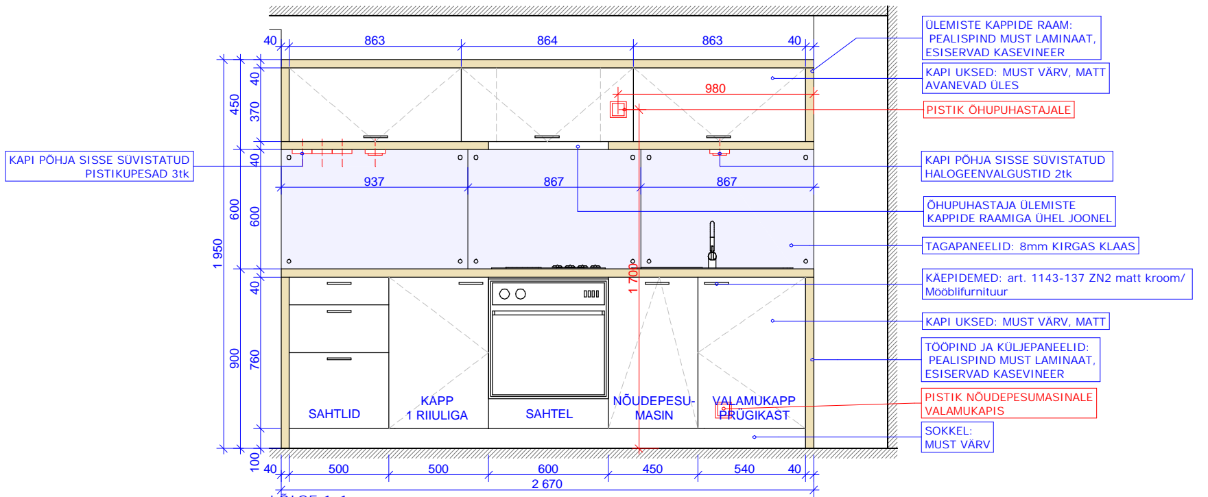
LÕIGE 1-1
