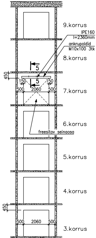
4-4 M1:100
