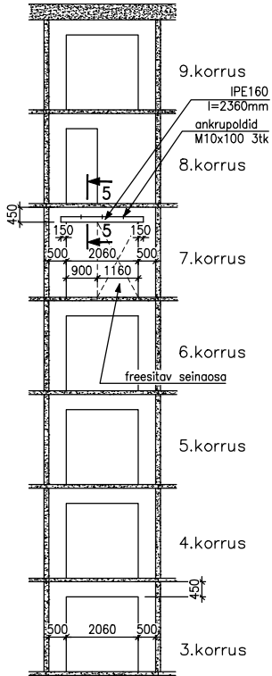
3-3 M1:100
