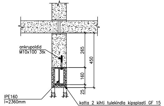
5-5 M1:10
