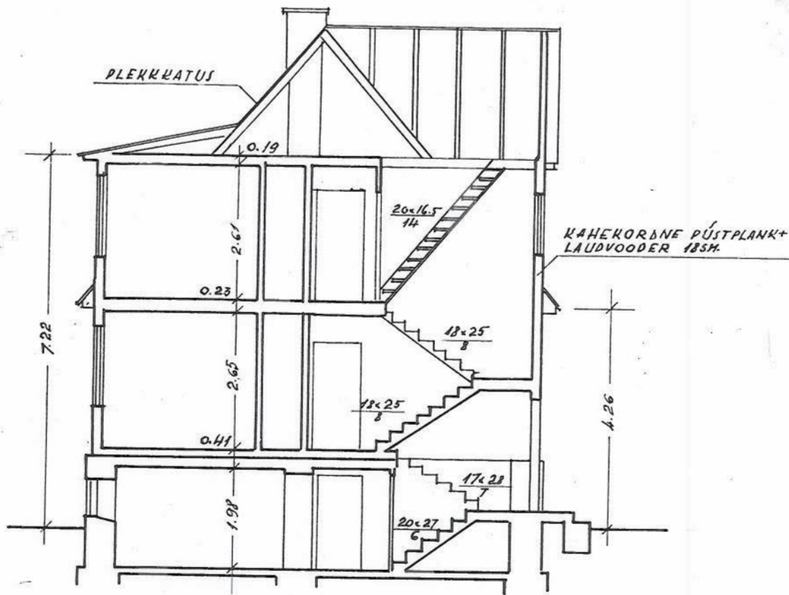
LÕIGE A-B
