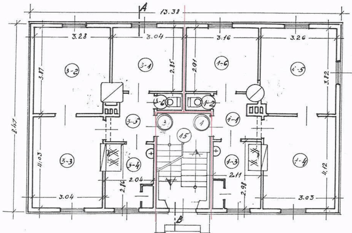
I KORRUS
