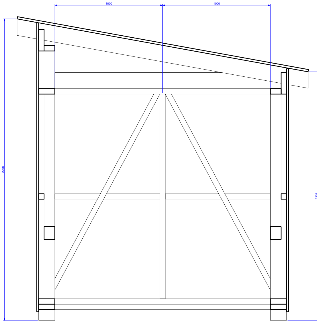
Lõige 1:20
