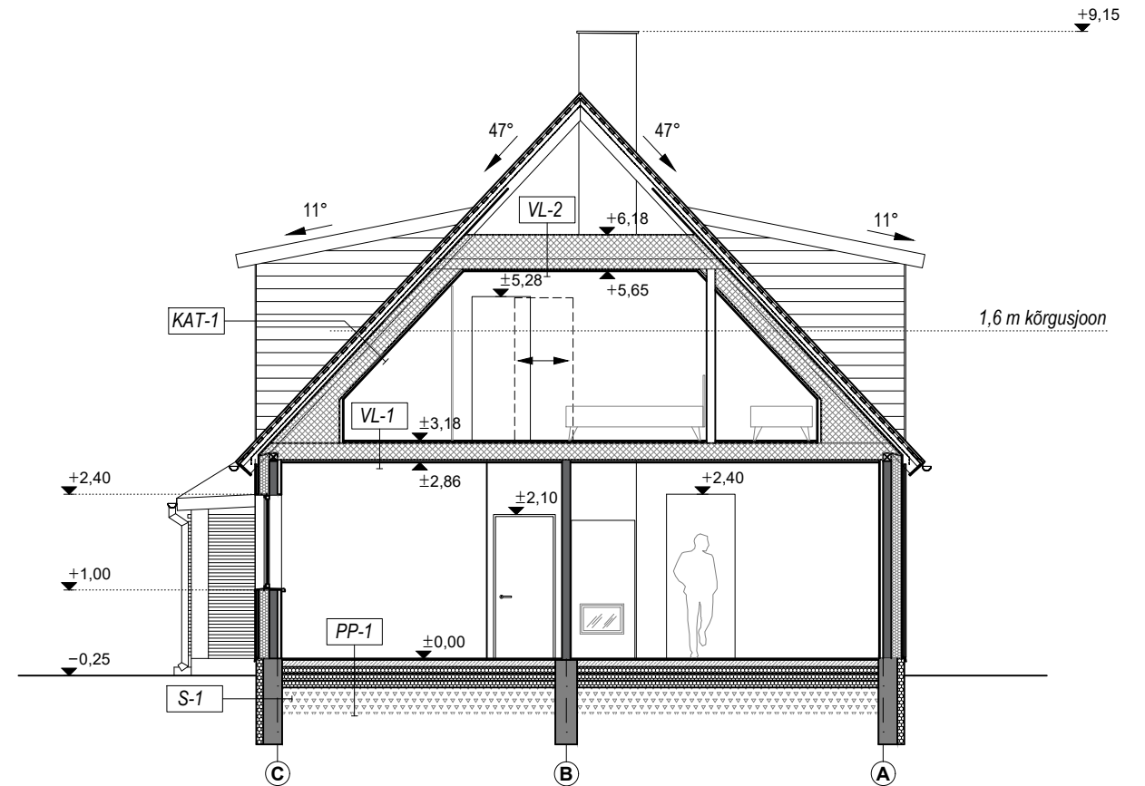
ELAMU LÕIGE 2-2 M 1:100
