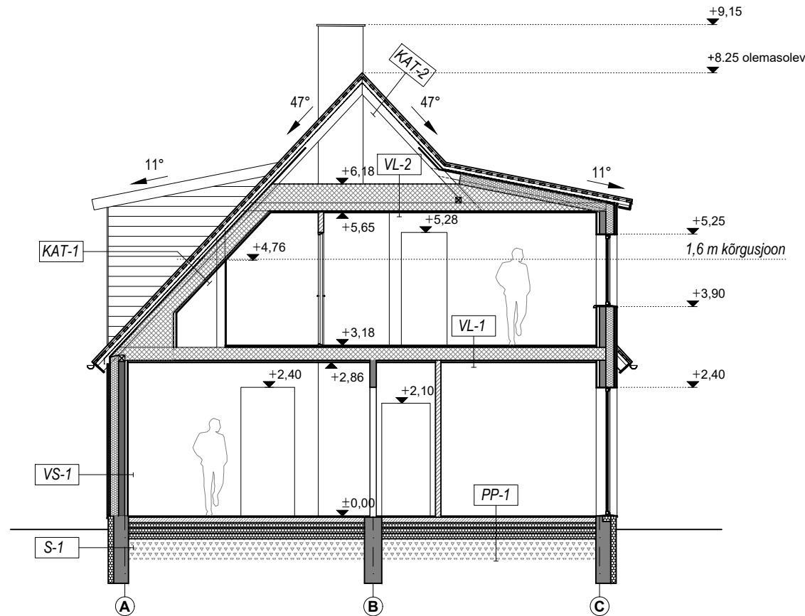
ELAMU LÕIGE 1-1 M 1:100
